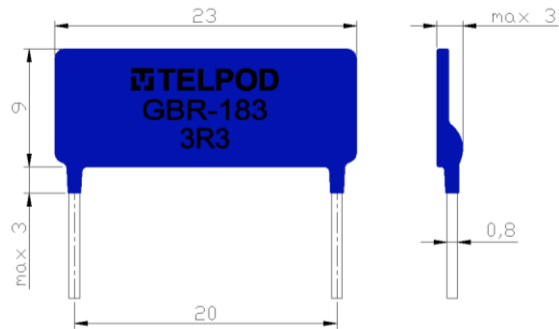
Abb. 1. Äußeres Erscheinungsbild und Abmessungen [mm]
